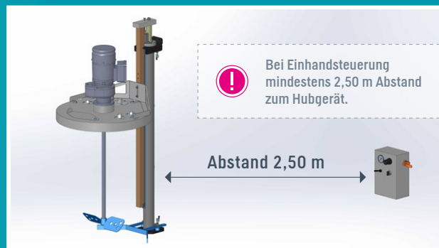
Rührstationen für 200 Liter Fässer
